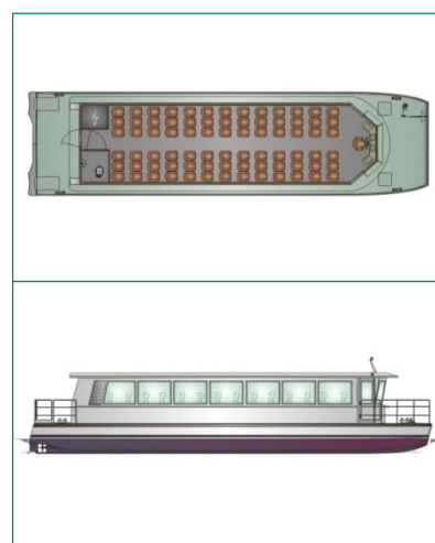
Fot. 14 Tramwaj wodny TW18 M. Źródło: http://www.tramwajwodne.pl/tw18.htm
