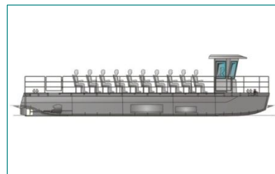
Fot. 16 Tramwaj wodny TW 150. Źródło: http://www.tramwajewodne.pl/tw20m.htm
